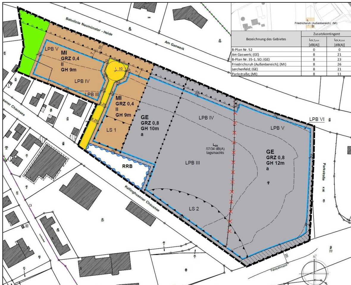
Abbildung 3: Bebauungsplan-Entwurf (Stand 15.02.2017)
